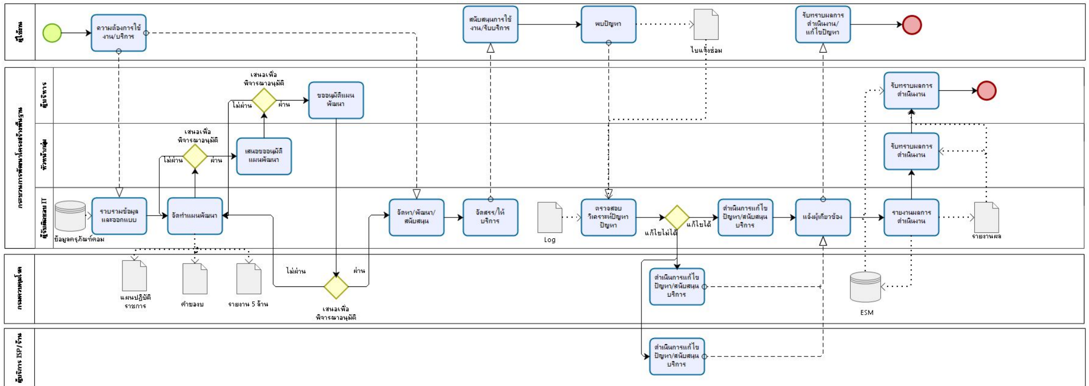
ตัวอย่าง BPMN กระบวนการ IT 1.พัฒนาโครงสร้างพื้นฐาน
